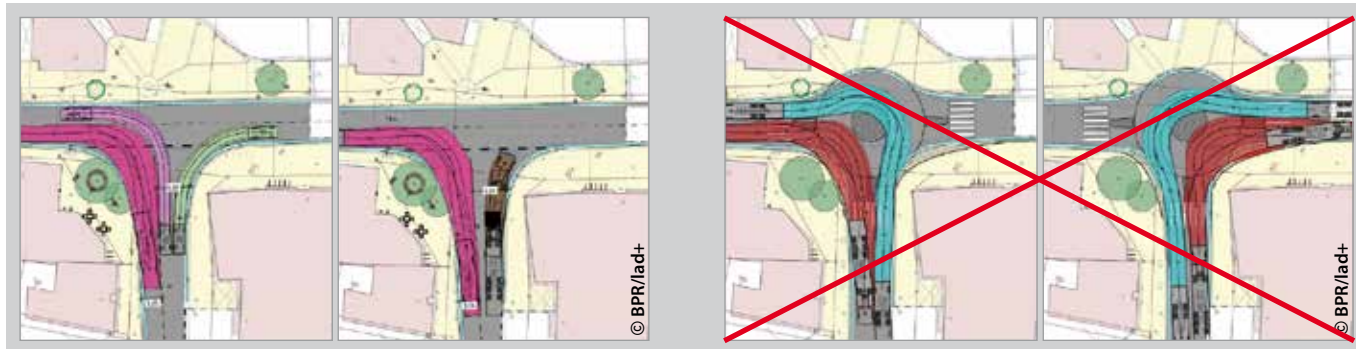
Der Ratsbeschluss sieht eine Erweiterung der vorhandenen Kreuzung vor (Abbildungen links). Abgelehnt wurde der von den Planern favorisierte Minikreisel mit 17 m Durchmesser (Abbildungen rechts).
